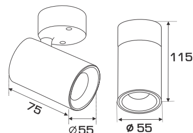
906D - Đèn Rây
