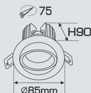
AFC 742 LED 7W 392.000
