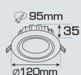
AFC 434 LED 9W 283.000 - 9W○○○3 chế độ sáng 354.000
